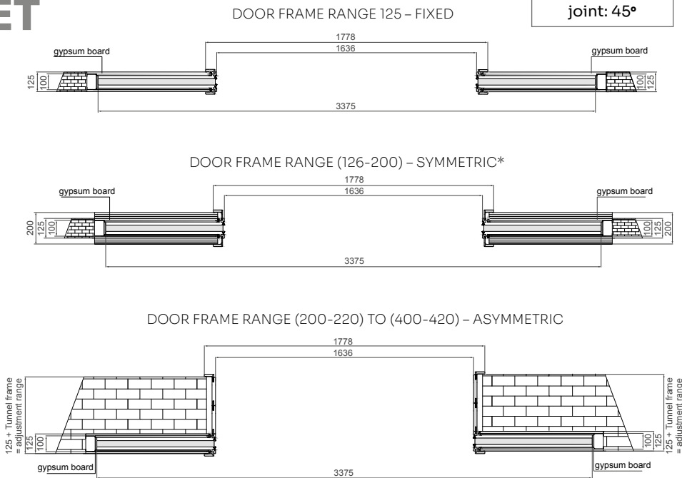
Door frame joint: 45°
